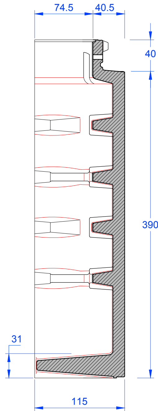
Schnitt A-A
