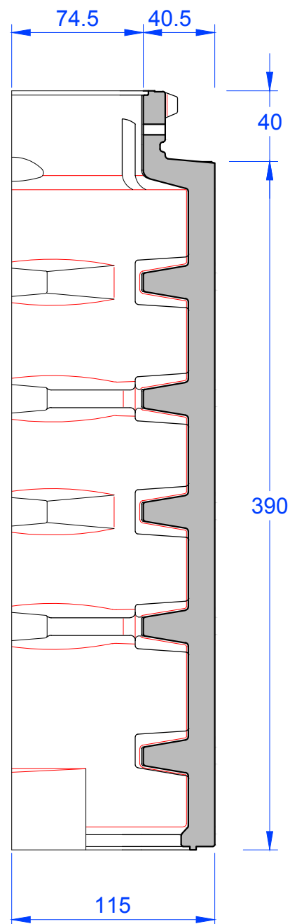
Schnitt A-A
