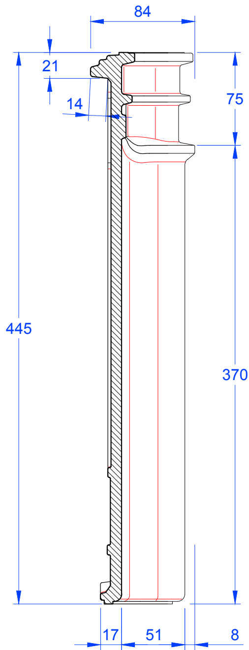
Schnitt B-B
