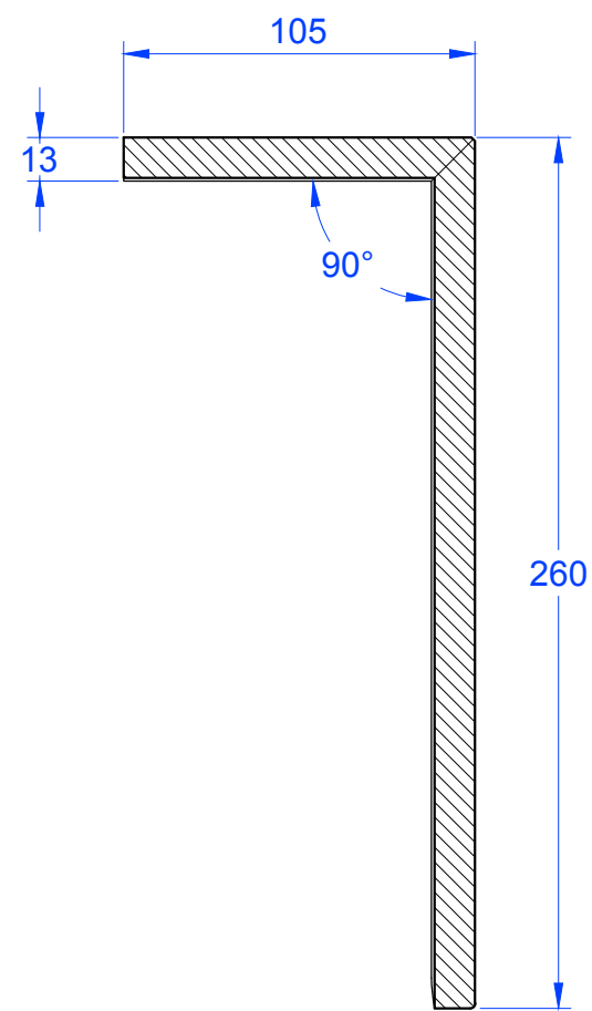
Schnitt B-B
