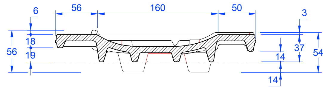
Schnitt A-A
