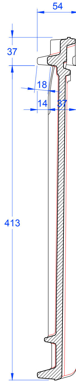
Schnitt B-B
