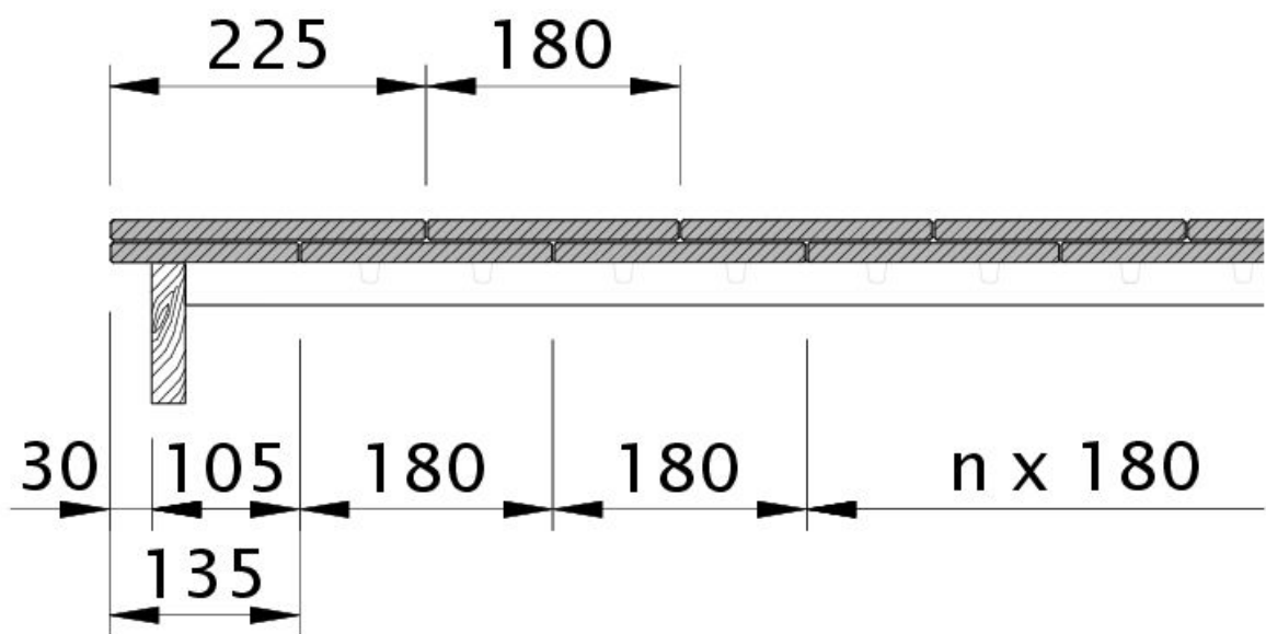
Zeichnung KLASSIK Orthgangziegel links mit Orthgangbrett und 1 1/4 Biber OBL114
