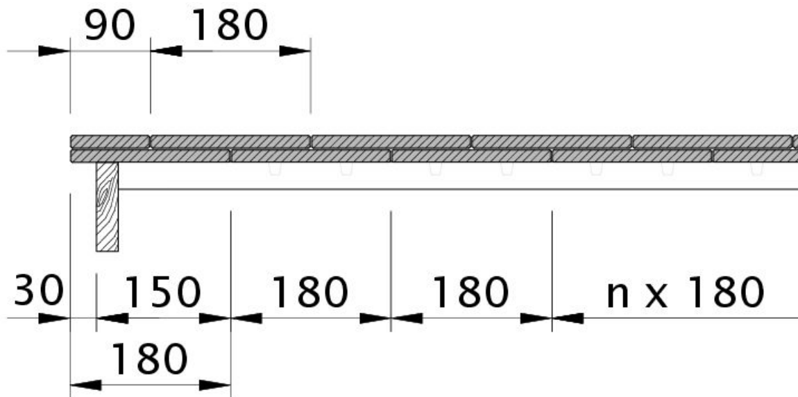
Zeichnung KLASSIK Orthgangziegel links mit Orthgangbrett und 1 1/2 Biber OBL112
