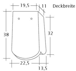
Zeichnung KLASSIK OG-1-1-4
